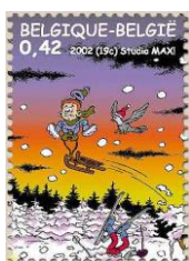
3103 sleeën
