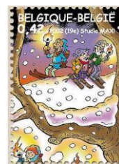
3105 Nachtskiën.
